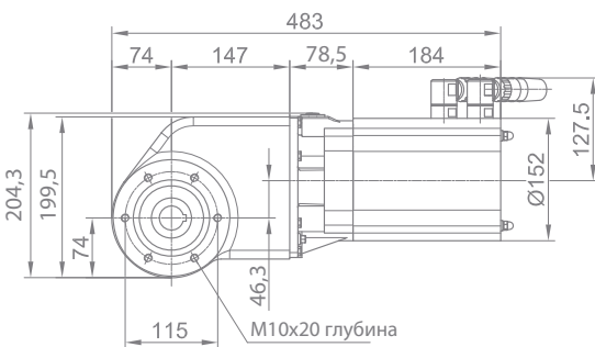
Габаритные размеры привода Danfoss VLT® OneGearDrive Hygienic™
